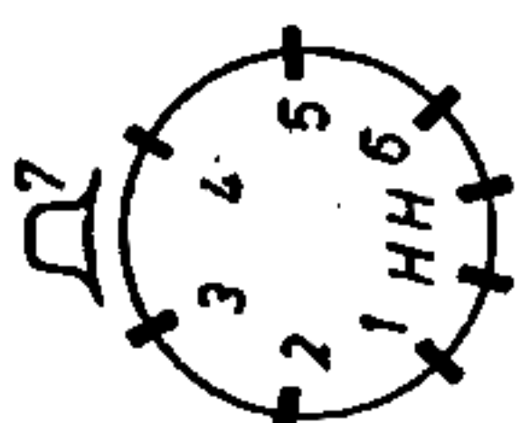
Socket/schaltung
